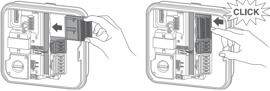
BAZ 4 İSTASYONLU MODÜL + PCM300 + PCM1600
