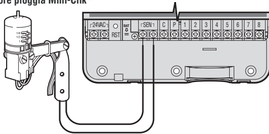
Sensore pioggia Mini-Clik®
