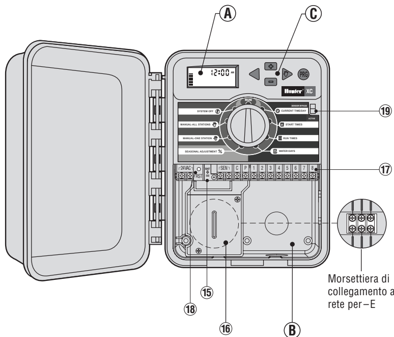
Modello per esterni (trasformatore interno incorporato)
