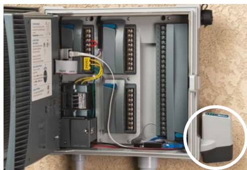
Controlador ICC2 com módulo LANKIT instalado
