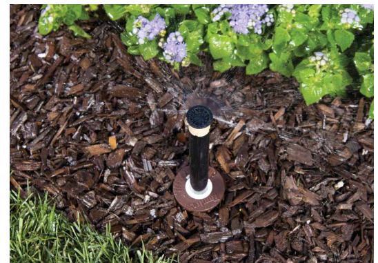
Kis sugarú mikroszóró fűvőka
